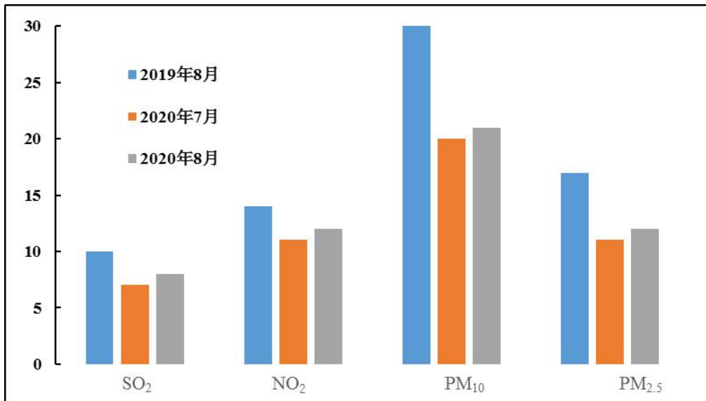
图1 云南省环境空气主要污染物月均值变化情况 (单位: µg/m³)
